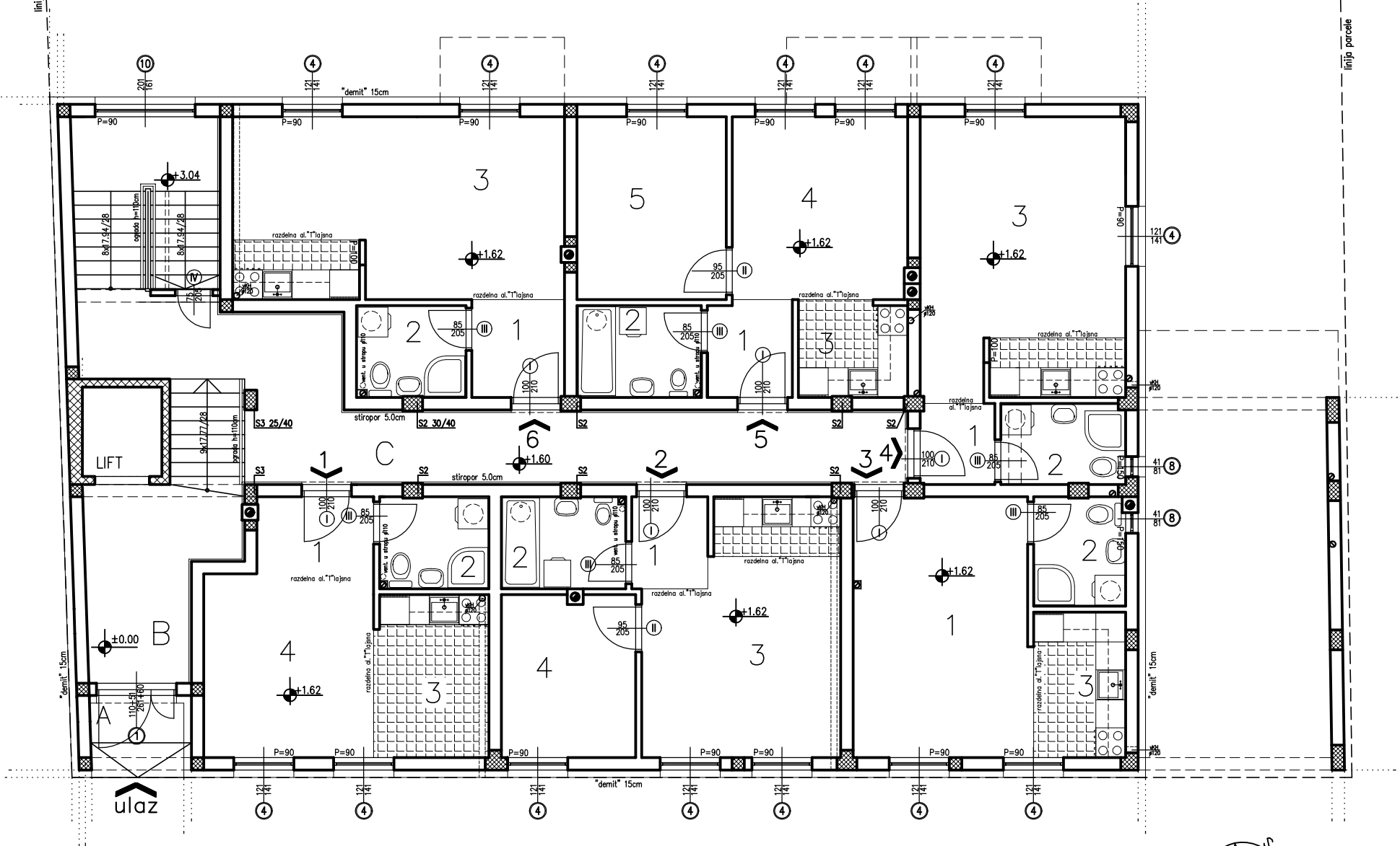
OSNOVA PRIZEMLJA 1:100
