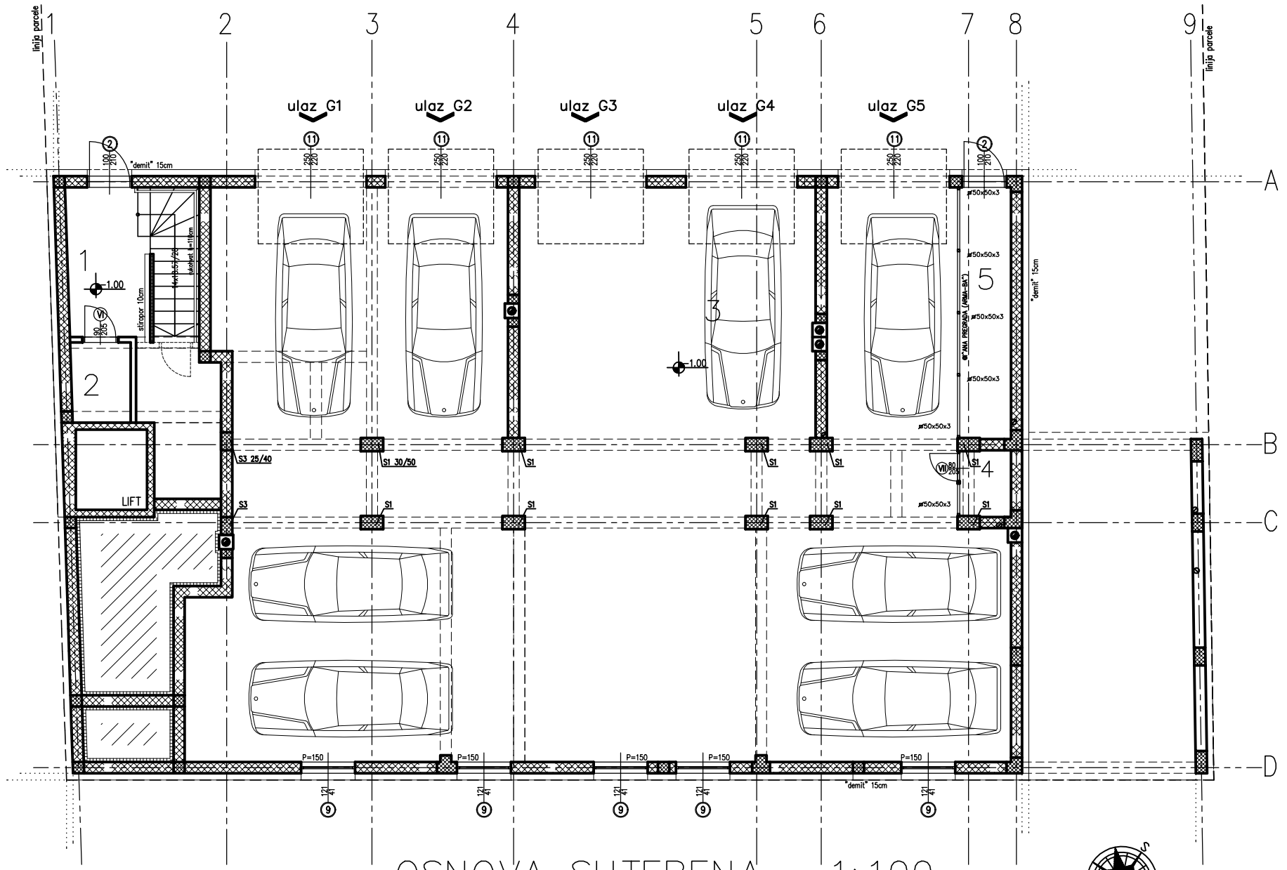
OSNOVA SUTERENA 1:100
